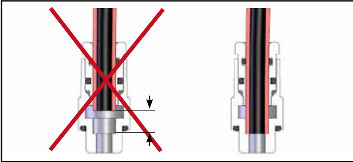
Bild 5: Einstecktiefe des Sensorschlauchs
